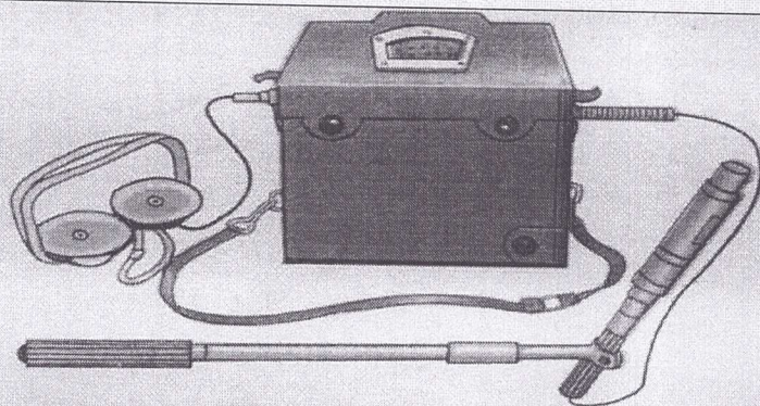
Прибор состоит из измерительного пульта 1 и зонда 2, соединенного с пультом гибким кабелем 3.
